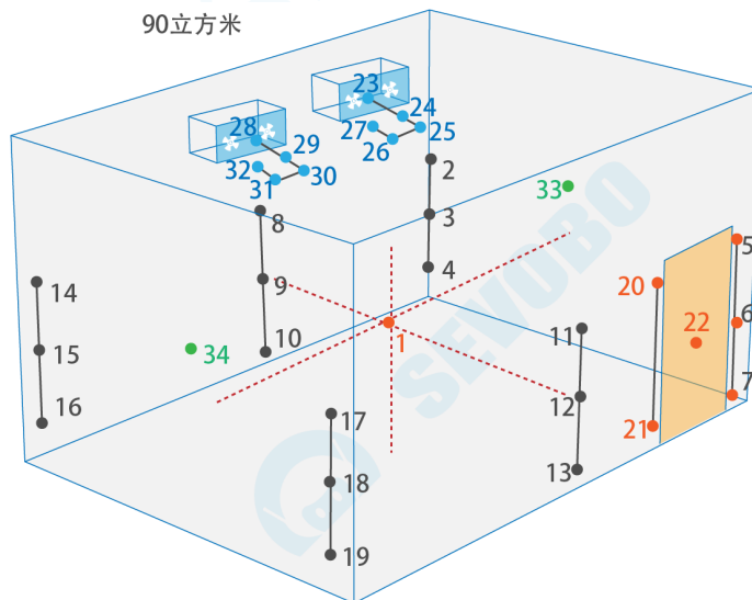
布点示意图
