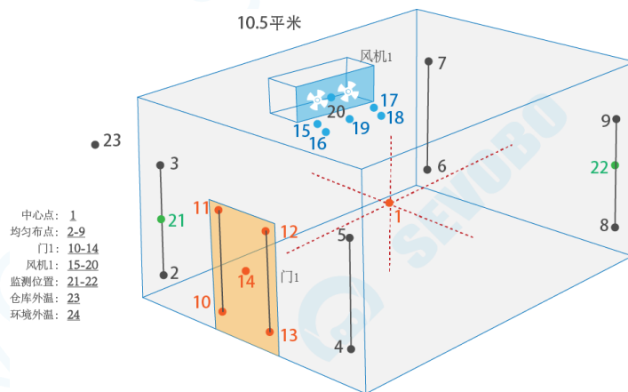
布点示意图
