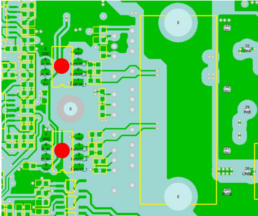
线路板的正面
