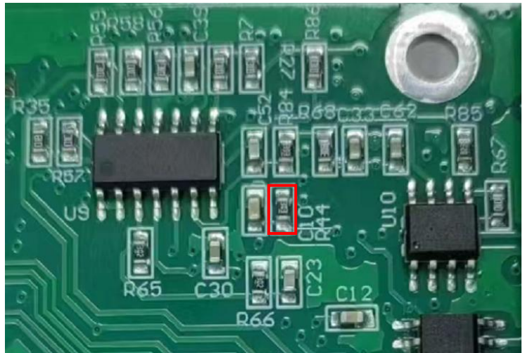
线路板背面
