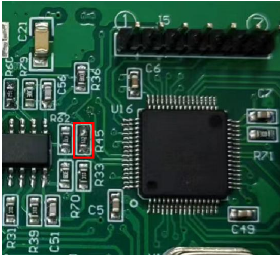
线路板的正面
