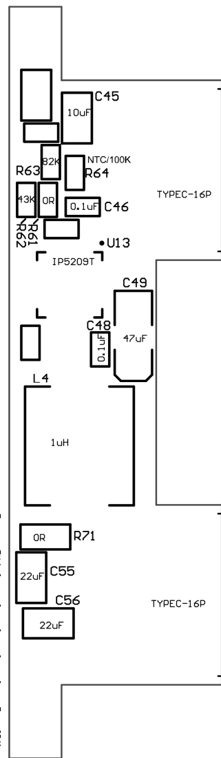
SVB-BT-4000-M_PCBA底层贴片图
