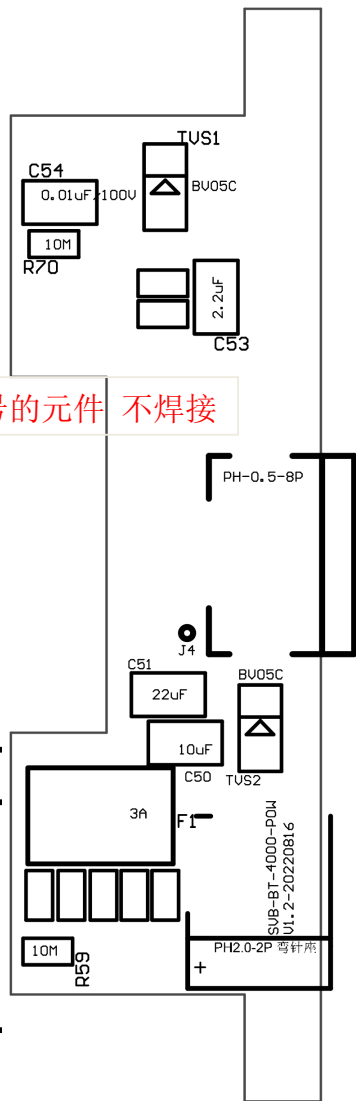
SVB-BT-4000-M_PCBA顶层贴片图
