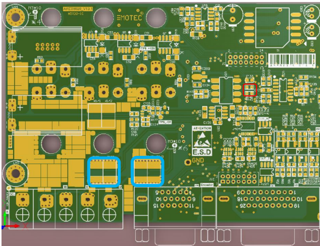
线路板正面
