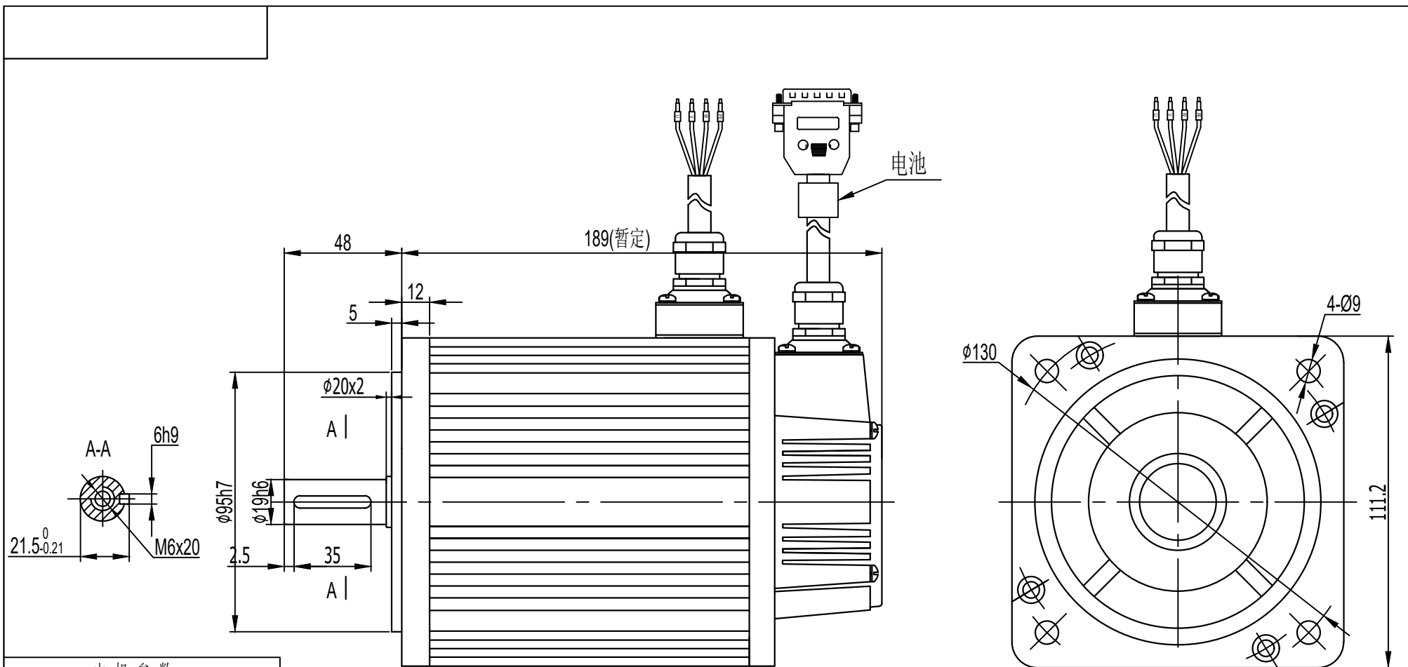
电机参数
