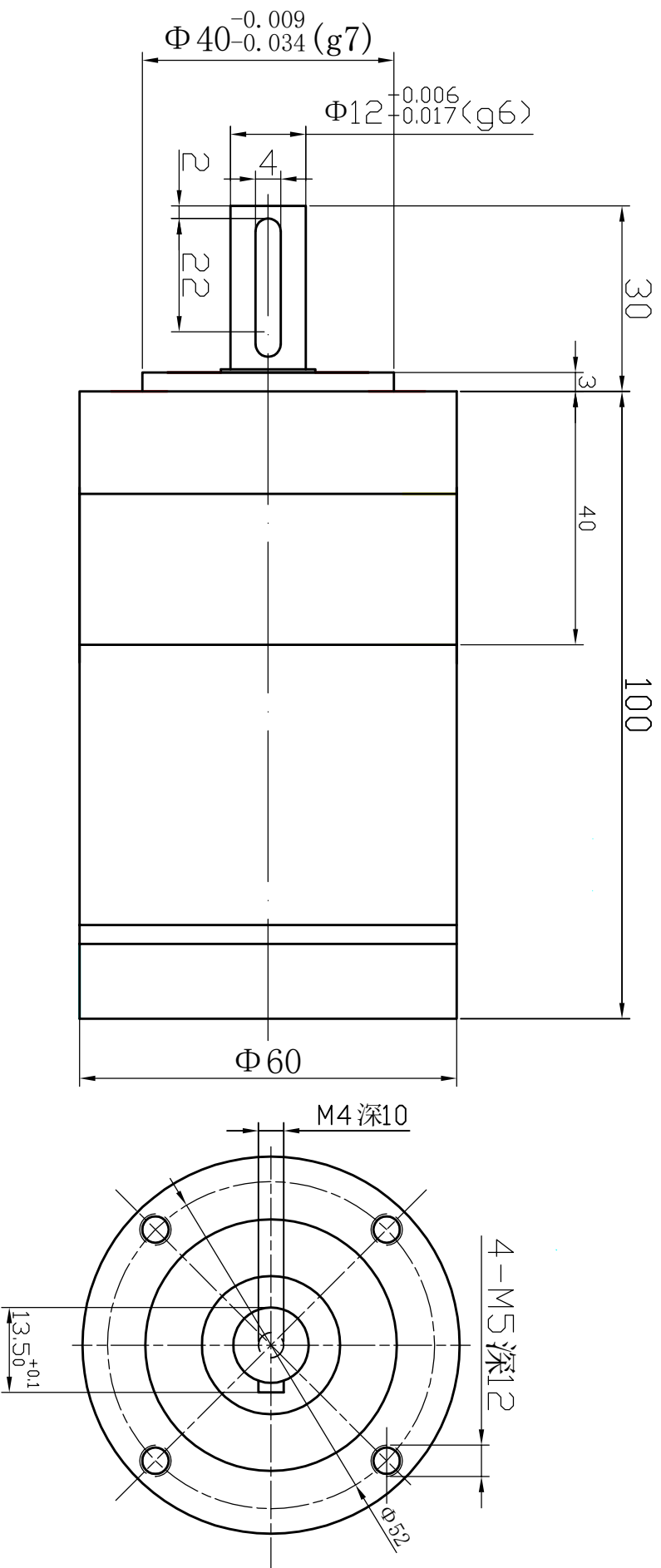
DSEM-G2460R055060N行星减速伺服直流电机外形图
